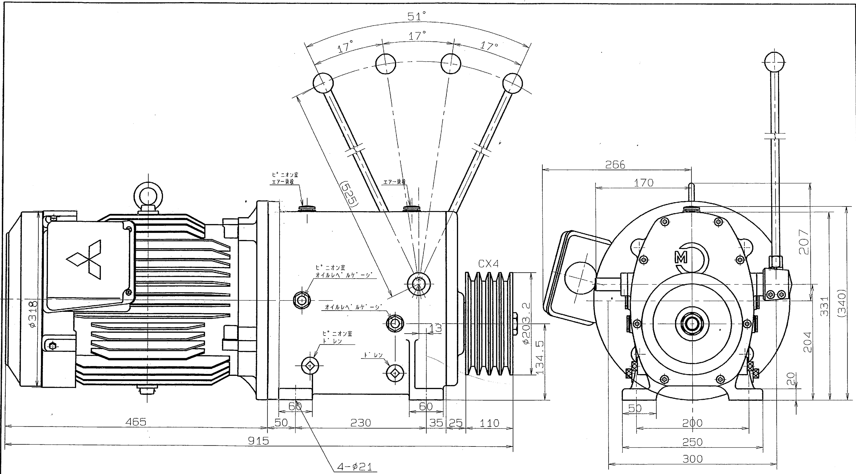
(MSD-410 6P外形図)
